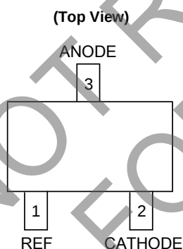
SOT-23
