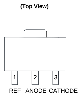
SOT-89 (Option 2)
