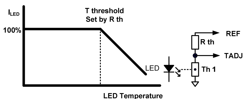
Fig. 4 Thermal control
