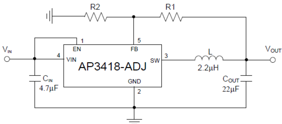
AP3418 SOT-23-5
